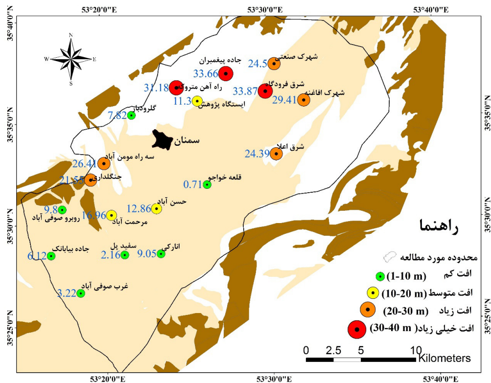
شکل ۳. پراکندگی پیژومترهای موجود در دشت و میزان افت کل در محل پیژومترها در طی ۲۴ سال مورد مطالعه
