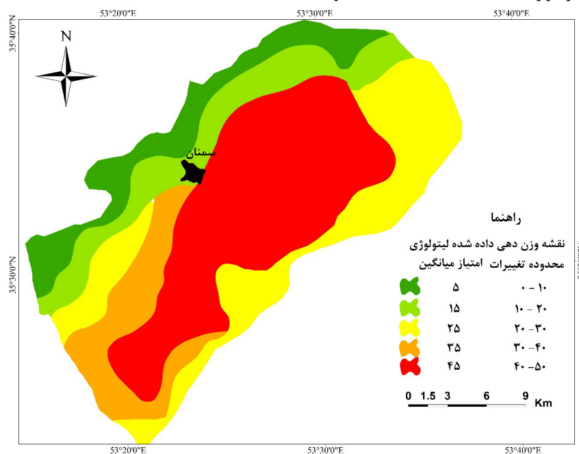
شکل ۱۰. نقشه زون‌بندی شرایط لیتولوژی دشت سمنان
