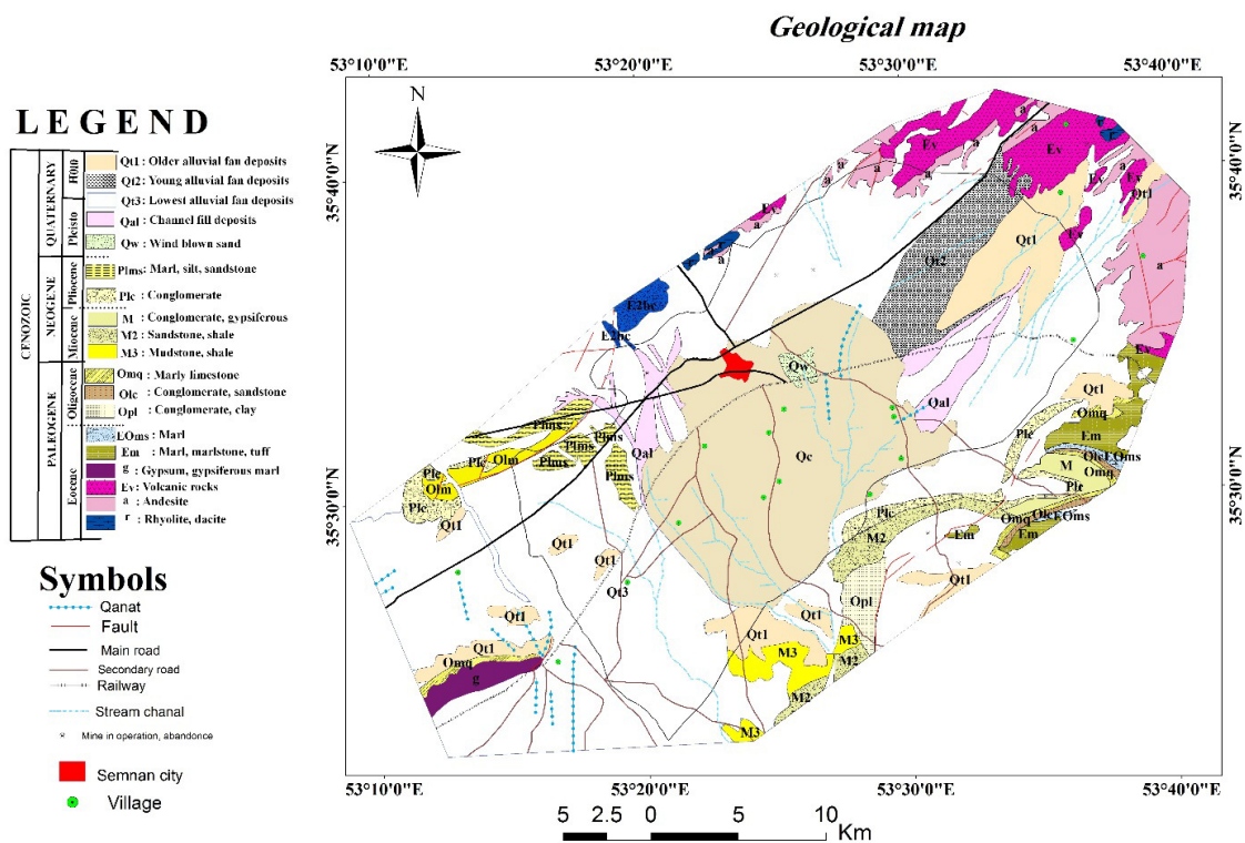
شکل ۲. نقشه زمین‌شناسی منطقه مورد مطالعه (برگرفته از نقشه زمین‌شناسی ۱/۲۵۰۰۰۰ سمnan (حدادان و همکاران، ۱۹۹۴)
